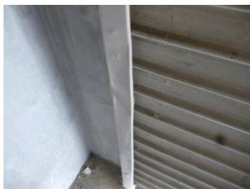
シャッター縦枠の変形
