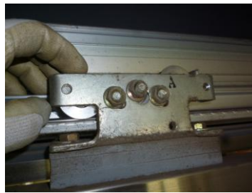
戸車調整
