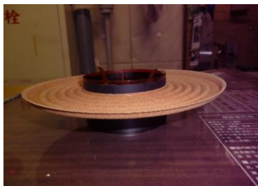
ボイスコイル・ダンパー仮組
