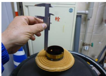
既存ボイスコイル取付位置合わせ
